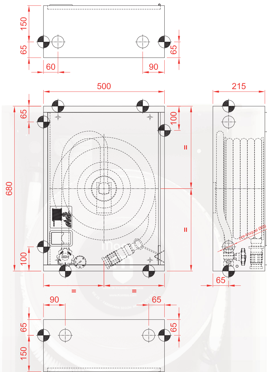
DIMENSIONES EMPOTRAMIENTO
