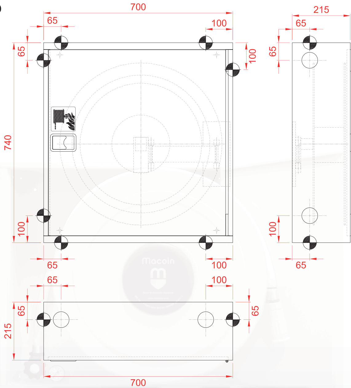
DIMENSIONES EMPOTRAMIENTO
